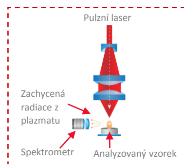
Schéma č. 2 – Princip technologie LIBS
